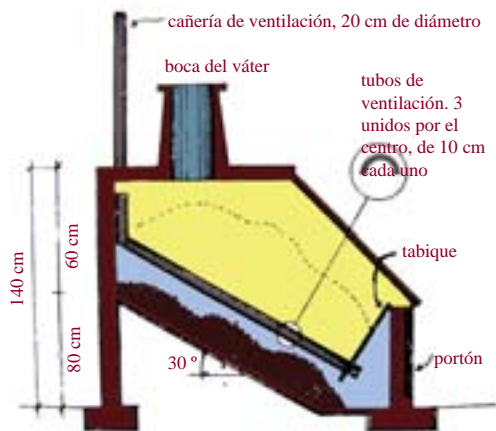
Esquema constructivo de un váter compostador Clivus.
